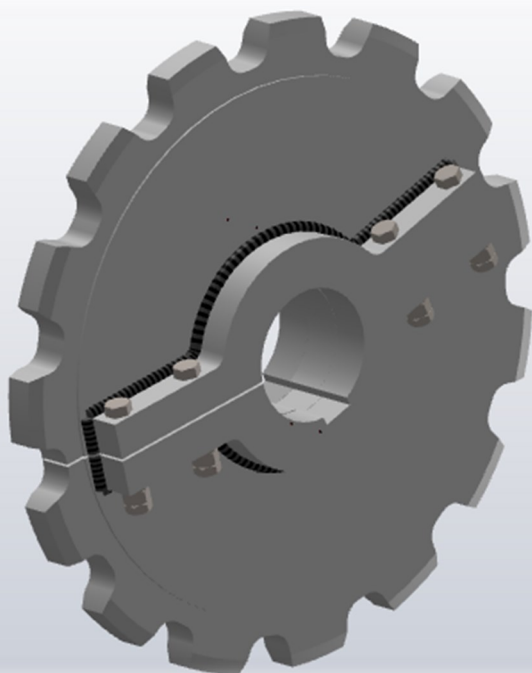
ENGRENAGEM BI-PARTIDA
